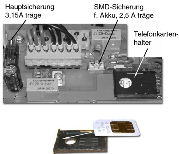
Abbildung 2: Telefonkarte einsetzen
