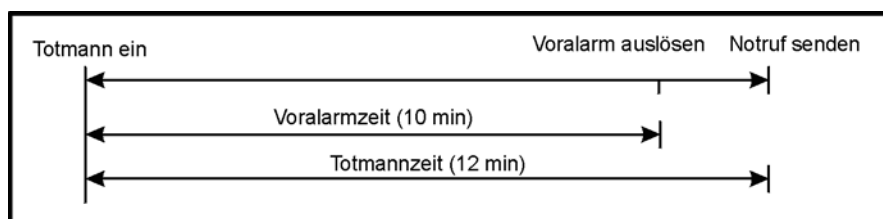
Abbildung 3: Totmannzeiten
